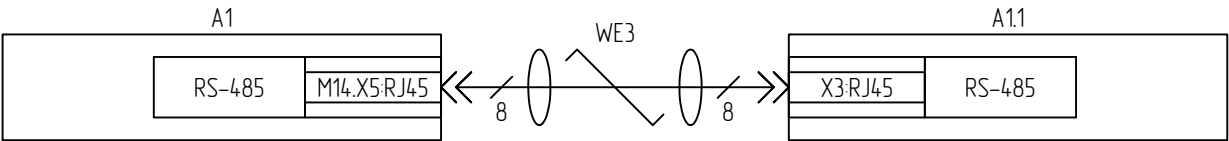
Цепи связи терминала с ИЧМ
