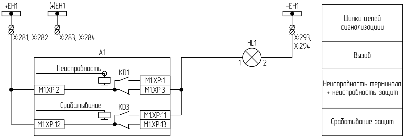
Цепи сигнализации А1
