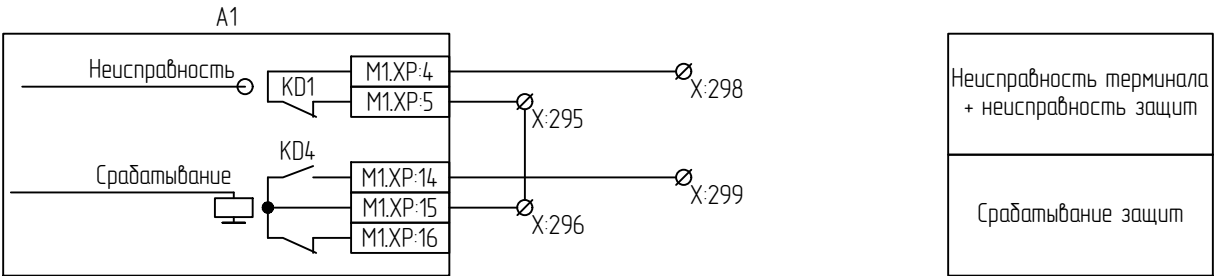
Цепи РАС А1
