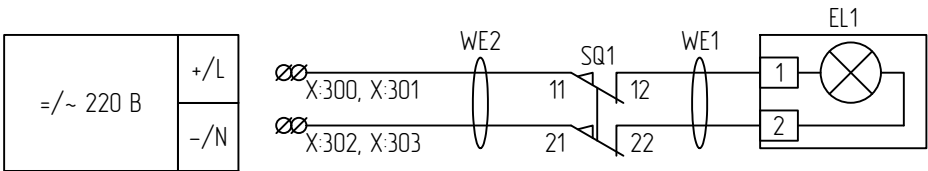
Цепи освещения шкафа
